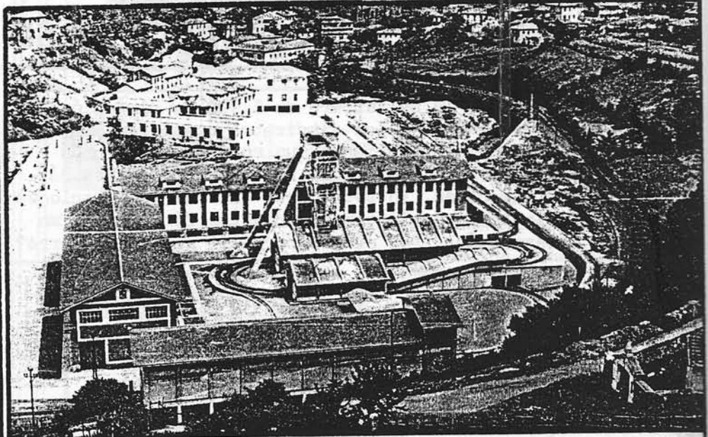
En primer plano, el Pozo San José, inaugurado oficialmente el 23 de septiembre de 1957. Tiene una profundidad de 430 metros (en explotación, 310 metros).
