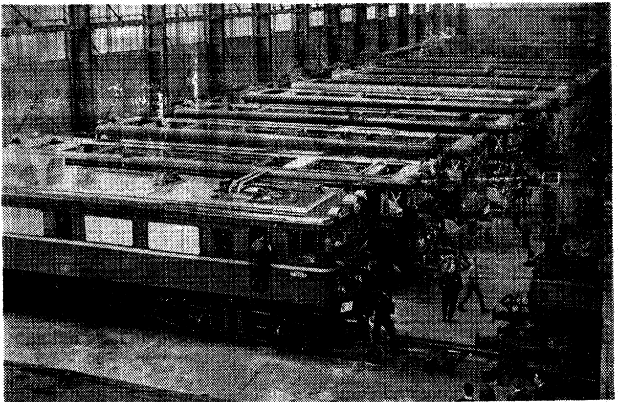
Vista del taller de montaje de la Compañía Auxiliar de Ferrocarriles de Beasain, donde se construyen locomotoras eléctricas, con licencia japonesa, de la marca «Mitsubishi». La primera locomotora, de una serie de 14, ha realizado ya sus pruebas oficiales antes de ser entregada a la R.E.N.F.E. Sus características son: 2.700 Kw. para tensión mixta de 1.500 y 3.000 voltios; velocidad máxima de 130 kilómetros por hora en trenes de viajeros y de 80 en los de mercancías; su peso es de 80 toneladas y su longitud, de tope a tope, de 17,270 metros. (Cifra)
